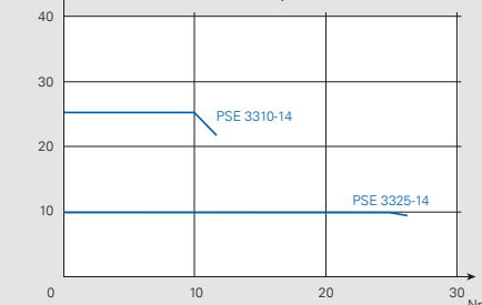
Kennlinie PSE 3310/3325-14
